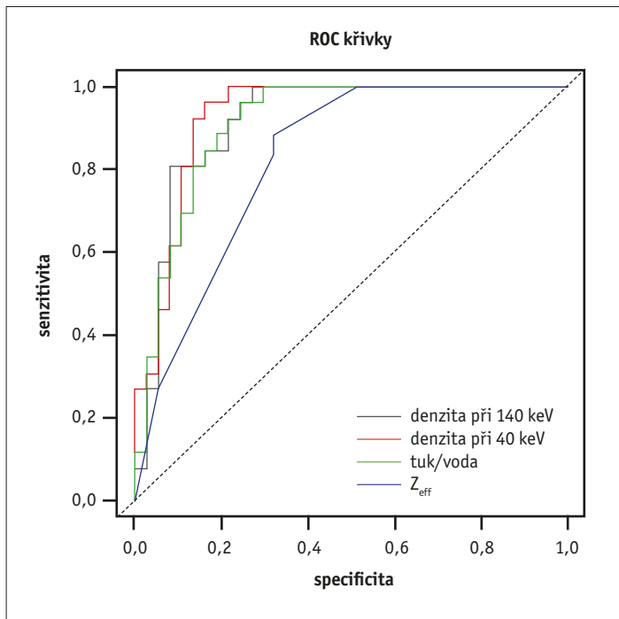
Graf 3. ROC křivky kvantitativních veličin
