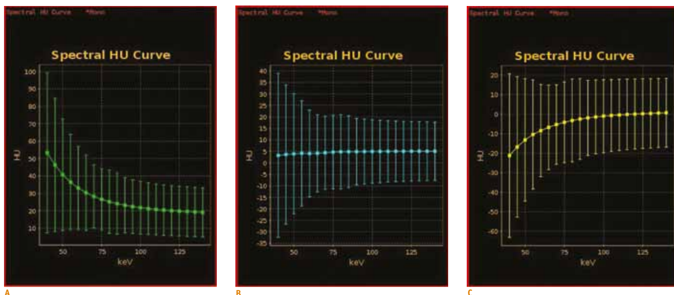
Graf 1. Příklady tří kategorií spektrálních křivek podle jejich průběhu: A – klesající, B – konstantní, C – stoupající Graph 1. Examples of three types of spectral HU curves according to their slope: A – descending, B – straight, C – ascending
