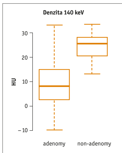
Graf 2. Krabicové grafy kvantitativních veličin vizuálně demonstrují statisticky významné rozdíly mezi adenomy a non-adenomy:
